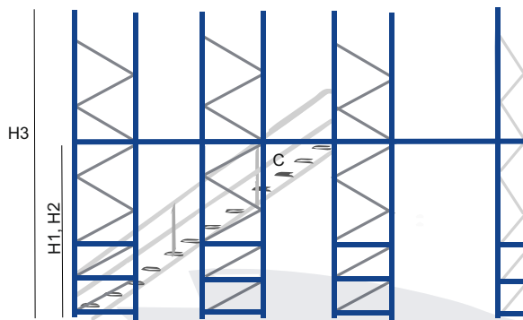
Мезонинная конструкция
